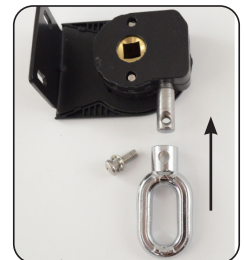
Instalación en el cielorraso
